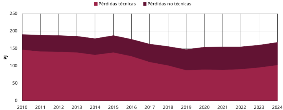
Figura 19. Figura 4.9 Evolución de las pérdidas energéticas, 2010-2024
